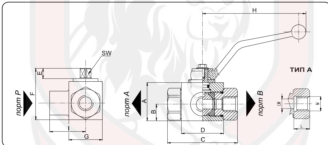
ТИП А : ПРИСОЕДИНИТЕЛЬНЫЙ КАНАЛ С ВНУТРЕННЕЙ ТРУБНОЙ РЕЗЬБОЙ ПО DIN/ISO 228 В SP
